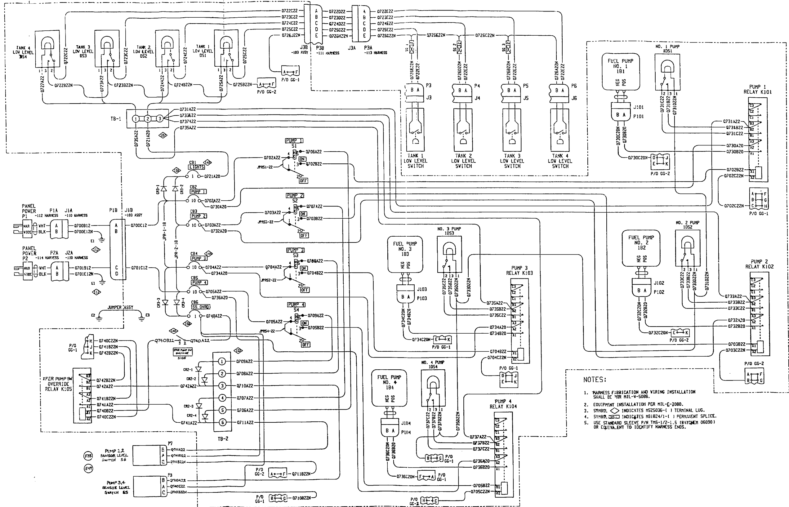
Figure FO-1. ERFS Wiring Diagram
